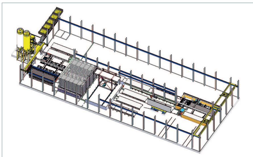
Схема расстановки компонентов линии с системой циркуляции поддонов
