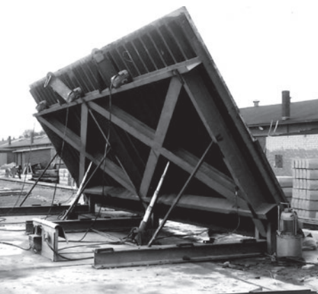
Konstrukcja stołu uchylnego z zamontowanymi ukośnymi stężeniami.
