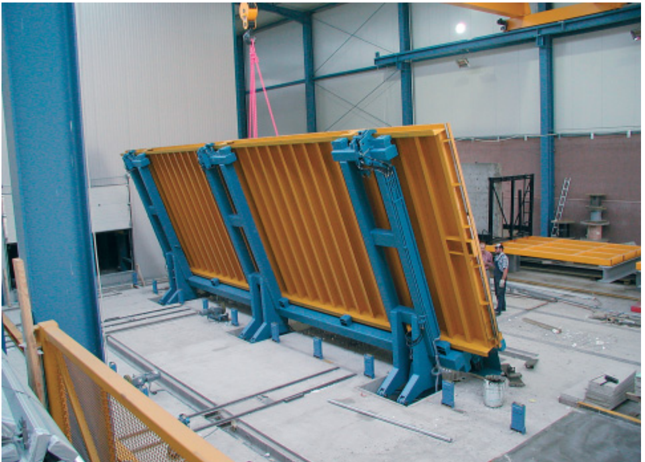
Kippstation mit Palettdurchfahrt in hoch gekippter Stellung zur Umlaufoptimierung
