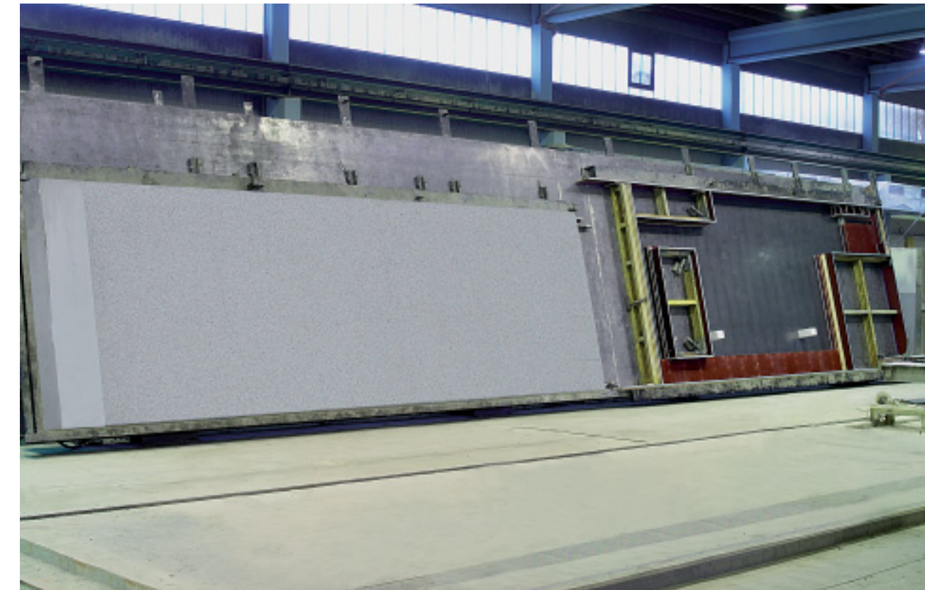
Hydraulischer Kipptisch
