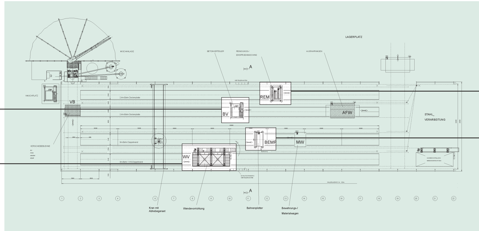
Produktionslayout einer automatisierten Bahnenfertigung für Elementdecken und Doppelwände
