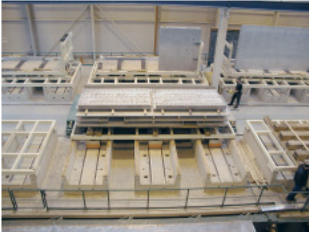
Ausfahrwagen in der Halle
