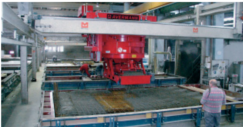
Betonverteiler mit Bandaustrag
